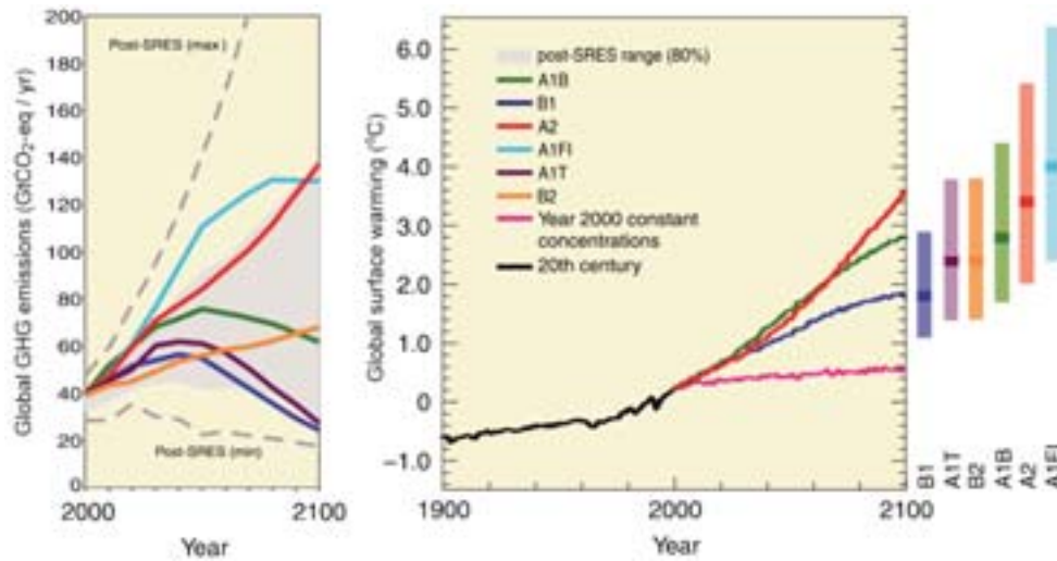
Slika 5. Lijevi prikaz: globalne emisije GHG-a (izražene u CO 2 -eq) u situaciji nepostojanja klimatskih politika; prikazuje šest ilustrativnih markerskih scenarija SRES (obojene linije) i raspon 80. percentila nedavnih scenarija objavljenih nakon SRES-a (post-SRES) (sivo obojeno područje). Isprekidane linije prikazuju puni raspon scenarija post-SRES. Emisije pokrivaju plinove CO 2 , CH 4 , N 2 O, i F. Desni prikaz: pune linije prikazuju višemodelne globalne prosjeke površinskog zagrijavanja za scenarije A2, A1B i B1 prikazane kao nastavak simulacije iz 20. stoljeća. Te simulacije uzimaju u obzir i emisije kratkotrajnih GHG-a i aerosola. Ružičasta linija ne prikazuje scenarij, već simulaciju modela opće cirkulacije između atmosfere i oceana (Atmosphere-Ocean General Circulation Model- AOGCM) u kojem su atmosferske koncentracije zadržane na razini iz 2000. godine. Stupići s desne strane slike prikazuju najbolje procjene (pune linije unutar svakog stupića) i vjerojatan raspon procijenjen za šest markerskih scenarija SRES za razdoblje 2090.—2099. godine. Sve su temperature izražene u odnosu na razdoblje 1980.—1999. godine. (slike 3.1 i 3.2)
