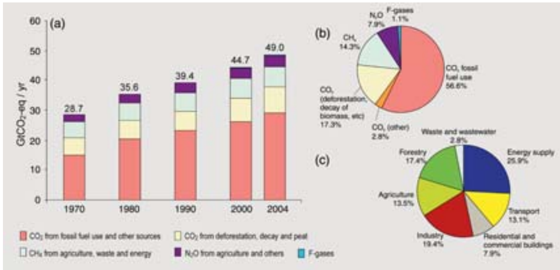
Slika 3. (a) Globalne godišnje emisije antropogenih GHG-a od 1970. do 2004. godine (b) Udio različitih antropogenih GHG-a u ukupnim emisijama u 2004. u smislu CO 2 -eq. (c) Udio različitih sektora u ukupnim emisijama antropogenih GHG-a u 2004. godini u smislu CO 2 -eq. (Šumarstvo obuhvaća krčenje šuma). {Slika 2.1}
