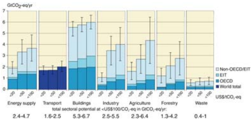
Slika 10. Procijenjen ekonomski potencijal ublažavanja prema sektorima u 2030. godini izražen na temelju studija bottom-up, uspoređen s odgovarajućim osnovama korištenima u ocjenjivanju sektora. Potencijali ne obuhvaćaju netehničke opcije kao što su promjene u stilu života. {Slika 4.2}
