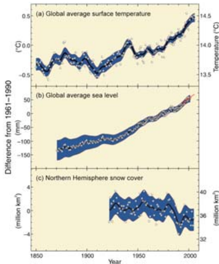
Slika 1. Opažene promjene (a) u globalno prosječnoj prizemnoj temperaturi; (b) u globalno prosječnom dizanju razine mora na temelju podataka dobivenih pomoću mareografa (plavo) i sa satelita (crveno), i u snježnom pokrovu na sjevernoj hemisferi od ožujka do travnja. Sve su promjene dane u odnosu na odgovarajuće prosjeke za razdoblje od 1961. do 1990. godine. Glatke krivulje prikazuju desetljetne uprosječene vrijednosti dok kružići prikazuju godišnje vrijednosti. Zasjenjena područja jesu intervali nesigurnosti dobiveni iz sveobuhvatne analize poznatih nesigurnosti (a i b) i iz vremenskih nizova (c). {slika 1.1}
