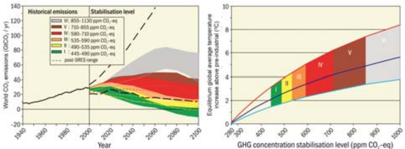
Slika 11. Globalne emisije CO 2 za razdoblje od 1940. do 2000. godine i rasponi emisija za kategorije stabilizacijskih scenarija od 2000. do 2100. godine (lijevi prikaz); i odgovarajući odnos između stabilizacijskog cilja i vjerojatnog ravnotežnog globalnog prosječnog povećanja temperature iznad pred-industrijske razine (desni prikaz). Približavanje ravnoteži može potrajati stoljećima, posebice za scenarije s visokim razinama stabilizacije. Obojena područja prikazuju stabilizacijske scenarije grupirane prema različitim ciljevima (stabilizacijske kategorije I do VI). Desni prikaz prikazuje raspone promjene globalne prosječne temperature iznad predindustrijske, koristeći (i) "najbolju procjenu" klimatske osjetljivosti od 3°C (crna linija u sredini obojenog područja), (ii) gornju granicu vjerojatnog raspona klimatske osjetljivosti od 4.5°C (crvena linija na vrhu obojenog područja) (iii) donju granicu vjerojatnog raspona klimatske osjetljivosti od 2°C (plava linija na dnu obojenog područja). Crne isprekidane linije na lijevom prikazu daju raspon emisija nedavnih osnovnih scenarija objavljenih nakon SRES-a (2000.). Rasponi emisija stabilizacijskih scenarija sadrže scenarije samo za CO 2 i scenarije za više plinova i odgovaraju 10. i 90. percintilu ukupne distribucije scenarija. Napomena: emisije CO 2 u većini modela ne uključuju emisije iz raspadanja nadzemne biomase koja ostaje nakon dobivanja trupaca i krčenja šuma, te iz požara tresetišta i isušenog tresetnog tla. {Slika 5.1}
