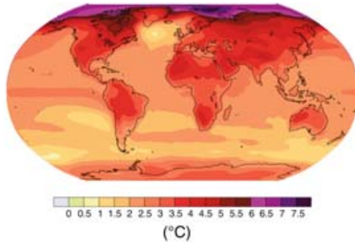
Slika 6. Projektirane promjene prizemne temperature za kraj 21. stoljeća (2090.—2099.). Karta pokazuje multi-AOGCM srednju projekciju za scenarij A1B SRES. Sve su temperature relativne u odnosu na razdoblje 1980.—1999. (slika 3.2)
