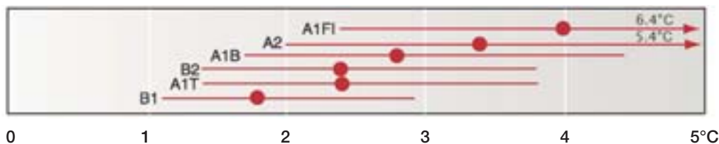
Slika 7. Primjeri utjecaja povezanih s očekivanim globalnim prosječnim prizemnim zagrijavanjem. Gornji prikaz: ilustrativni primjer globalnih utjecaja predviđenih za klimatske promjene (odnosi se i na razinu mora i atmosferski CO 2 gdje je relevantno) povezane s različitim povećanjima globalne prosječne prizemne temperature u 21. stoljeću. Crna linija povezuje utjecaje; isprekidane strelice ukazuju na utjecaje koji traju uz povećanje temperature. Podaci su upisani tako da lijeva strana teksta ukazuje na približnu razinu zagrijavanja koja je povezana s početkom danog utjecaja. Kvantitativni podaci za nedostatak vode i poplave predstavljaju dodatne utjecaje promjene klime u odnosu na uvjete predviđene nizom SRES-scenarija A1 F1, A2, B1 i B2. U tim procjenama nije uzeta u obzir prilagodba promjeni klime. Razina sigurnosti u sve te izjave visoka je. Donji prikaz: točkica i stupići prikazuju najbolju procjenu i vjerojatni raspon zagrijavanja procijenjen za šest markerskih scenarija SRES za razdoblje 2090.—2099. u odnosu na razdoblje 1980.—1999. godine {Slika 3.6}
