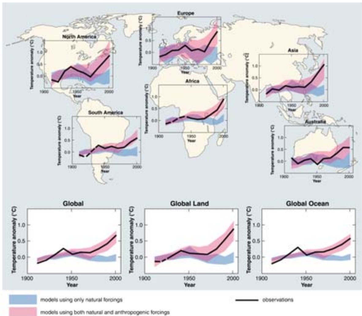
Globalna i kontinentalna promjena temperature
