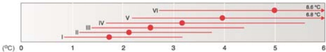
Promjena globalne prosječne temperature u odnosu na razdoblje 1980.—1999.
