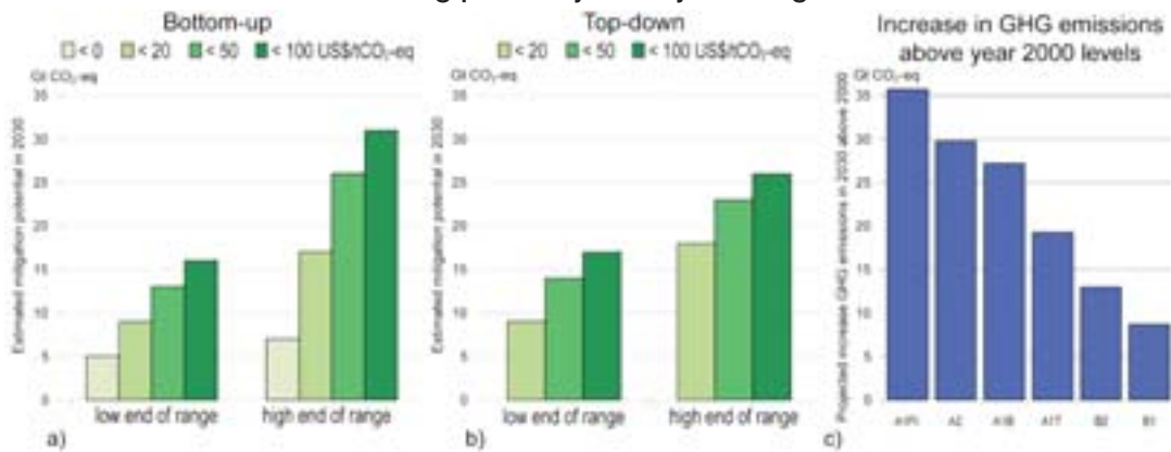
Slika 9. Globalni ekonomski potencijal ublažavanja u 2030. godini procijenjen na temelju studija bottom-up (Prikaz a) i top-down (Prikaz b), uspoređen s očekivanim povećanjima emisija iz SRES-scenarija u odnosu na emisije GHG-a od 40,8 GtCO 2 -eq (Prikaz c) iz 2000. godine.
