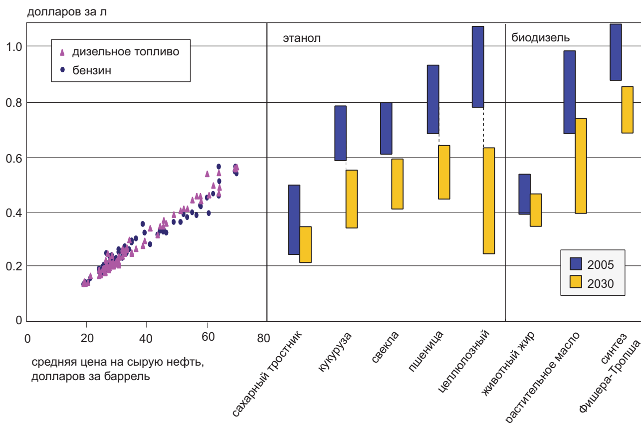
Рис. TS.16. Сравнение текущих и будущих затрат на производство биотоплива в сравнении с заводскими ценами (ФОБ) на бензин и дизельное топливо в диапазоне цен на сырую нефть [Figure 5.9].
