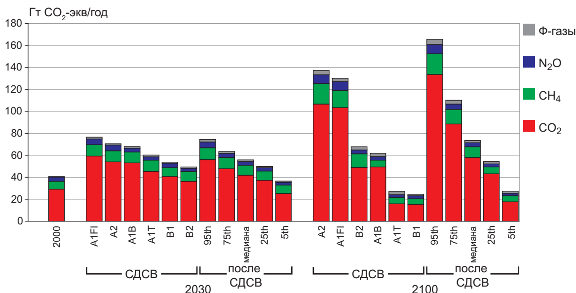
Рис. SPM 4. Глобальные выбросы ПГ для 2000 и прогнозируемые базовые выбросы на 2030 и 2100 годы по СДСВ и по литературе, вышедшей после СДСВ. На рисунке показаны выбросы по шести иллюстративным СДСВ сценариям. Он также даёт представление о плотности распределения выбросов по сценариям после СДСВ (5-й, 25-й, срединный, 75-й, 95-й процентиль), как показано в главе 3. Ф-газы включают ХФУ, ГФУ и SF6 [1.3, 3.2, рис. 1.7]. [примечание редактора: нижние индексы в легенде]
