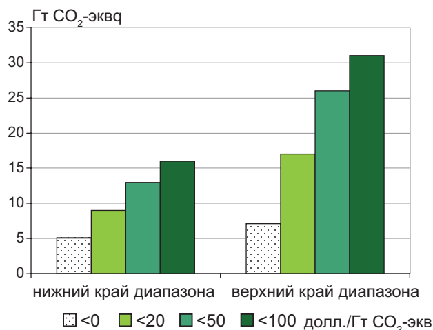
Рис. SPM 5A: Глобальный экономический потенциал в 2030 году по оценкам из восходящих исследований (данные из табл. SPM 1)
