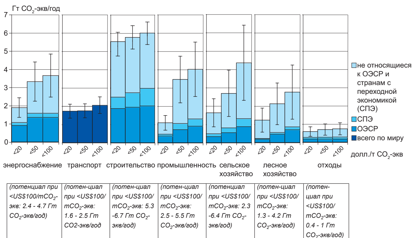
Рис. SPM 6: Предполагаемый отраслевой экономический потенциал глобального смягчения по разным регионам, как функция цены углерода в 2030 году по восходящим исследованиям, в сравнении с соответствующими базовыми цифрами, принятыми в отраслевых оценках. Полное объяснение построения этого рисунка приведено в п. 11.3.
