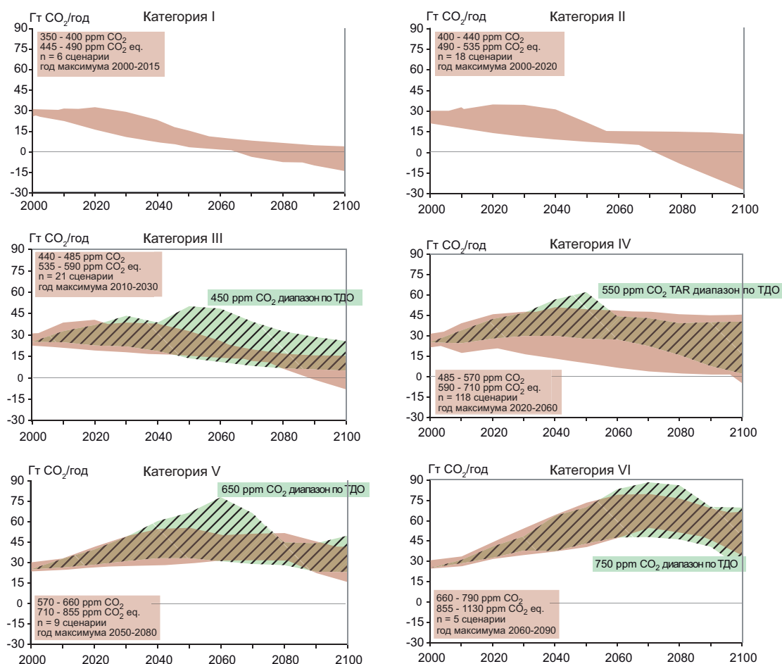
Рис. TS.8. Траектории выбросов по сценариям смягчения для альтернативных категорий уровней стабилизации (Категория с I по VI, как определено в вставке в каждой панели). Светло-коричневые области означают выбросы \text{CO}_2 для последних сценариев выбросов после ТДО. Зелёные и заштрихованные области означают диапазон более чем 80 сценариев стабилизации по ТДО (Morita et al., 2001). В сценариях по категории I и II изучаются цели по стабилизации ниже минимального уровня по ТДО. Выбросы за базисный год могут отличаться по моделям вследствие различий в охвате секторов и отраслей промышленности. Для достижения более низких уровней стабилизации некоторые сценарии предусматривают удаление \text{CO}_2 из атмосферы (отрицательные выбросы) с использованием таких технологий, как производство энергии из биомассы с использованием улавливания и хранения углерода. [Figure 3.17]
