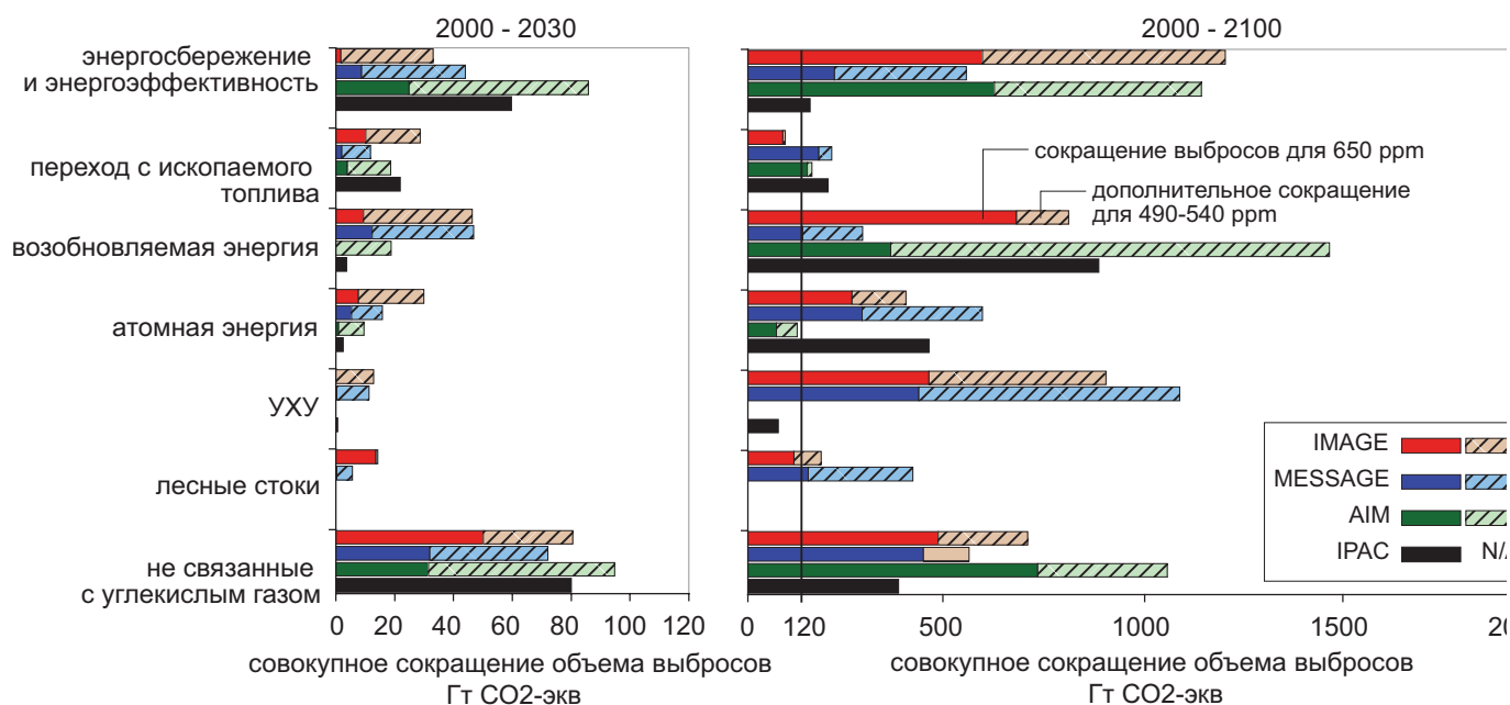
Рис. SPM 9. Совокупное снижение выбросов для альтернативных мер по смягчению последствий на 2000-2030 гг. (левая панель) и на 2000-2100 гг. (правая панель). На рисунке показаны иллюстративные сценарии из четырёх моделей (AIM, IMAGE, IPAC и MESSAGE), целью которых является стабилизация до 490-540 ppm CO 2 -экв и до уровней 650 ppm CO 2 -экв, соответственно. Тёмные полосы обозначают снижение для цели 650 ppm CO 2 -экв, а светлые – дополнительное снижение для достижения уровня 490-540 ppm CO 2 -экв. Отметим, что в некоторых моделях не учитывается смягчение последствий посредством расширения лесных стоков (AIM и IPAC) или УХУ (AIM) и что доля возможностей энергетики с низкой углеродоёмкостью в общей структуре энергоснабжения также определяется включением этих инструментов в базовые условия. УХУ включает улавливание и хранение углерода из биомассы. Лесные стоки включают сокращение выбросов от обезлесения. [Figure 3.23]]
