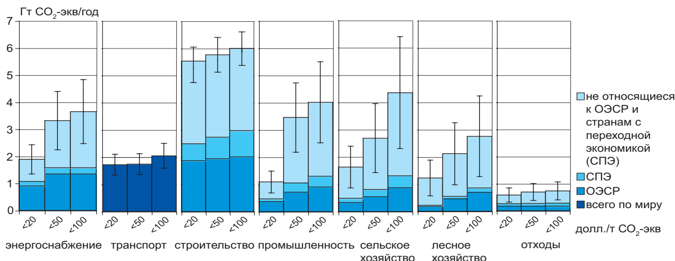
Рис. TS.27. Оценка экономического потенциала глобального смягчения по секторам и различным регионам как функция цены углерода в 2030 году по данным восходящих исследований в сравнении с соответствующими базовыми уровнями, предположенными в оценках по секторам. Полное объяснение получения этого рисунка приведено в п. 11.3.
