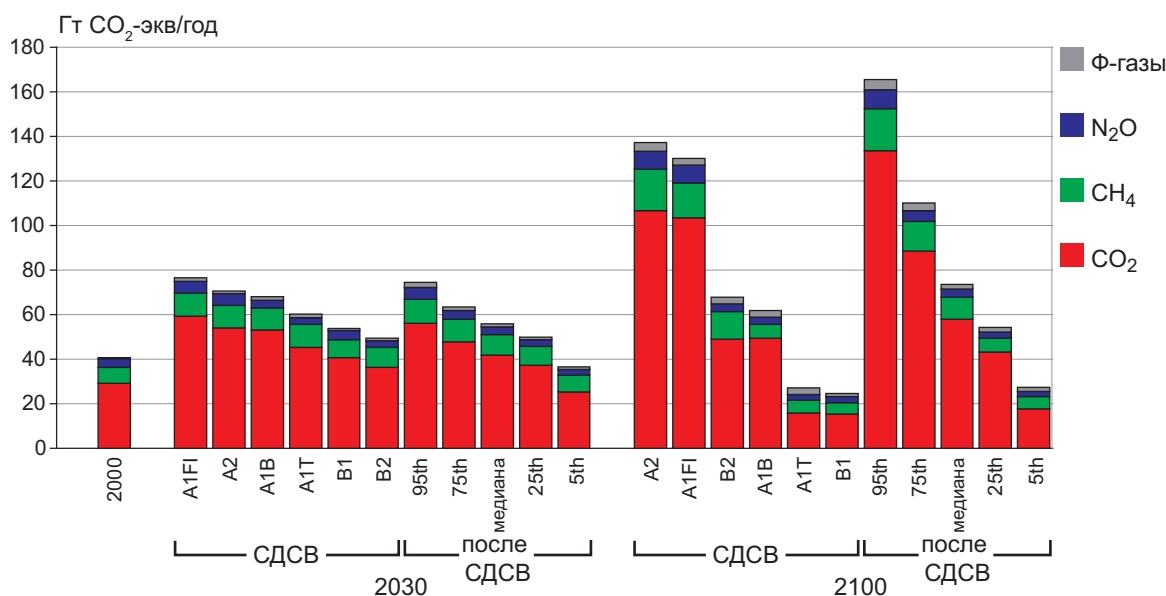
Рис. TS 5. Глобальные выбросы ПГ за 2000 г. и проекции базовых выбросов на 2030 и 2100 годы по СДСВ и по литературе, вышедшей после СДСВ. На рисунке показаны выбросы по шести иллюстративным сценариям СДСВ. Он также даёт представление о плотности распределения выбросов по сценариям после СДСВ (5-й, 25-й, срединный, 75-й, 95-й процентиля), как показано в главе 3. Ф-газы включают ХФУ, ГФУ и SF 6 [Figure 1.7].
