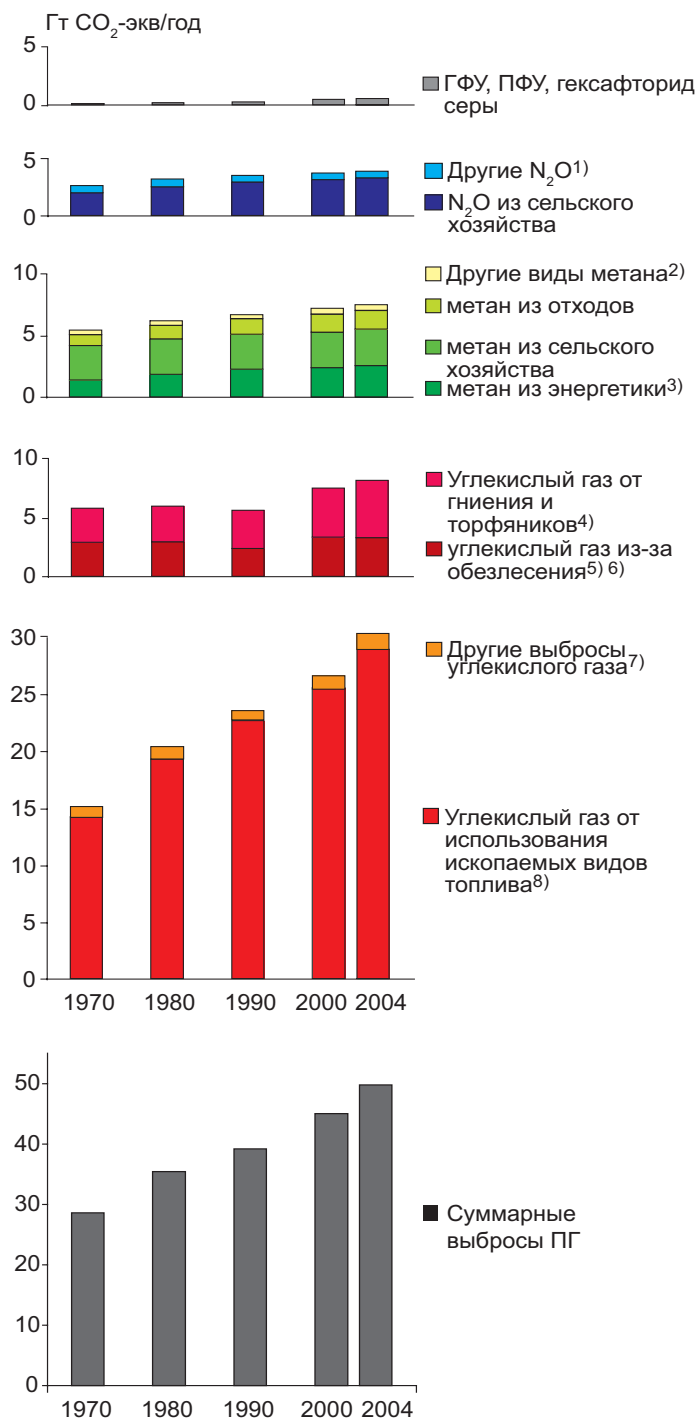
Рис. SPM 1. Глобальные выбросы парниковых газов, взвешенные по потенциалу глобального потепления (ПГП), за 1970-2004 годы. Для преобразования выбросов в эквивалент углекислого газа использовались 100-летние ПГП из доклада МГЭИК за 1996 год (ВДО) (ср. руководящие принципы отчетности по РКИК ООН). Включены CO 2 , CH 4 , N 2 O, ХФУ, ПФУ и SF 6 из всех источников. Две категории выбросов CO 2 отражают выбросы от производства и потребления энергии (второй график сверху) и от изменений в землепользовании (третий график сверху) [рис. 1.1a].
