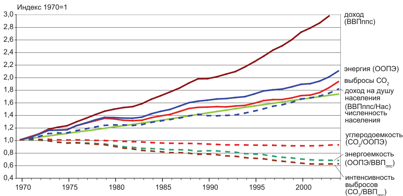
Рис. SPM 2. Относительное глобальное развитие внутреннего валового продукта, рассчитанного на основе ППС (ВВП ппс ), общего объема первичной энергии (ООПЭ), выбросов CO 2 (от сжигания ископаемого топлива, сгорания природного газа и производства цемента) и численности населения (Нас). Кроме того, пунктирными линиями на рисунке показаны доход на душу населения (ВВП ппс /Нас), энергоёмкость (ООПЭ/ВВП ппс ), углеродоемкость энергоснабжения (CO 2 /ООПЭ), и интенсивность выбросов в процессах экономического производства (CO 2 /ВВП ппс ) за период 1970-2004 гг. [рис. 1.5]
