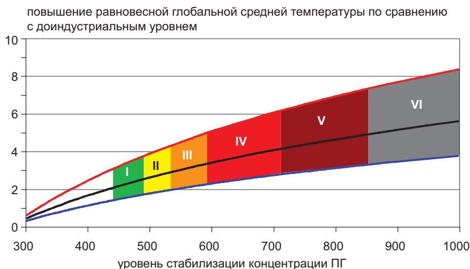
Рис. SPM 8: Категории сценариев стабилизации, как показано на Рис. SPM.7 (цветные полосы) и их связь с изменением равновесной глобальной средней температуры по сравнению с доиндустриальным уровнем. Использованы: (1) «наилучшая оценка» чувствительности климата 3°C (черная линия посередине закрашенной области); (2) верхняя граница вероятного диапазона чувствительности климата 4,5°C (красная линия, ограничивающая закрашенную область сверху); (3) нижняя граница вероятного диапазона чувствительности климата 2°C (синяя линия, ограничивающая закрашенную область снизу). Закрашенная область обозначает диапазоны концентрации для стабилизации парниковых газов в атмосфере, соответствующие категориям сценариев стабилизации I–VI, показанным на рис. SPM.7. Данные взяты из ДО4 РГІ, глава 10.8.
