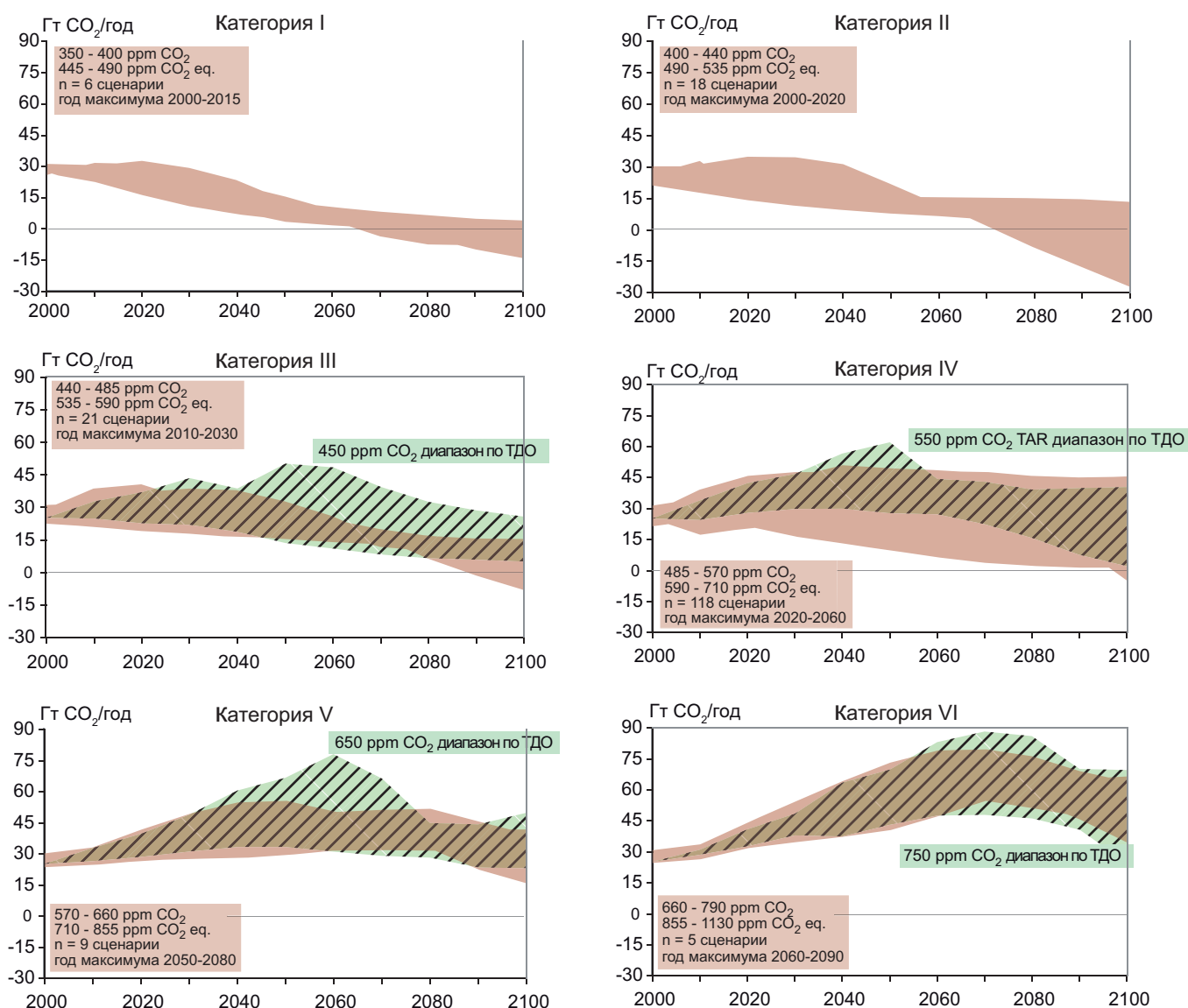
Рис. SPM 7. Траектории выбросов по сценариям смягчения для альтернативных категорий уровней стабилизации (Категория с I по VI, как определено во вставке в каждой панели). Траектории показаны только для выбросов CO 2 . Светло-коричневые области означают выбросы CO 2 для сценариев выбросов после ТДО. Зелёные области означают диапазон более чем 80 сценариев стабилизации по ТДО. Выбросы за базовый год могут отличаться по моделям в зависимости от отличий в охвате секторов и отраслей промышленности. Для достижения более низких уровней стабилизации некоторые сценарии предусматривают удаление CO 2 из атмосферы (отрицательные выбросы) с использованием таких технологий, как производство энергии из биомассы с использованием улавливания и хранения углерода. [Figure 3.17]
