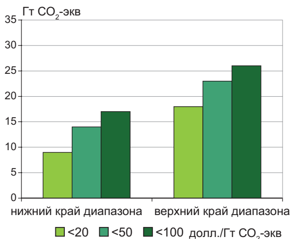
Рис. SPM 5B: Глобальный экономический потенциал в 2030 году по оценкам из нисходящих исследований (данные из табл. SPM 2)
