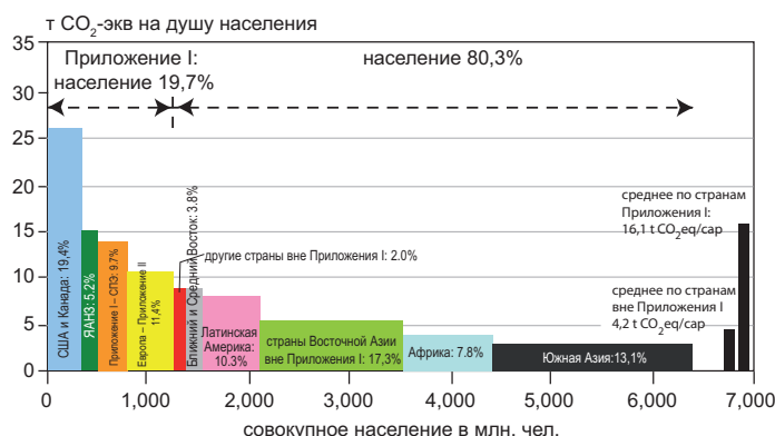
Рис. SPM 3а. Распределение региональных выбросов ПГ на душу населения в 2004 году (все газы Киотского протокола, включая и те, которые обусловлены землепользованием) по населению различных групп стран. Проценты в столбиках означают долю регионов в глобальном объеме выбросов ПГ [рис. 1.4а].
