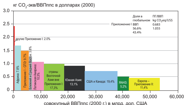
Рис. SPM 3б. Распределение региональных выбросов ПГ (все газы Киотского протокола, включая и те, которые обусловлены землепользованием) в 2004 г. на доллар США ВВП ппс к ВВП ппс для различных групп стран. Проценты в столбиках означают долю регионов в глобальном объеме выбросов ПГ [рис. 1.4б].
